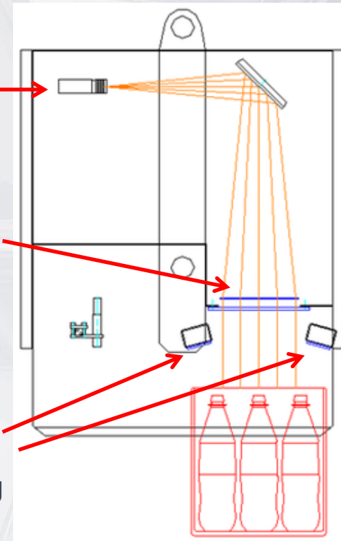
LK Querschnitt
